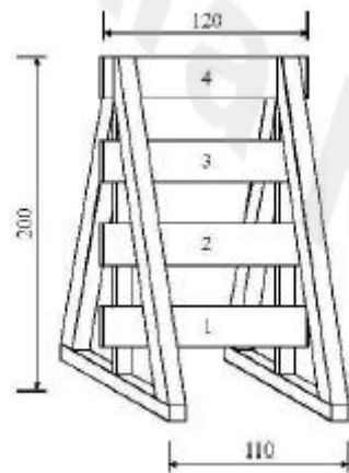
FIGURA b - ȘTACHETĂ - Tronson 5
