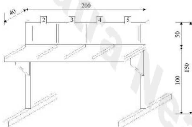
FIGURA e - RASTEL PENTRU NODURI
