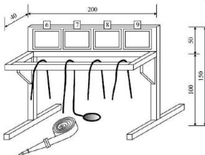
FIGURA e - RASTEL PENTRU NODURI
